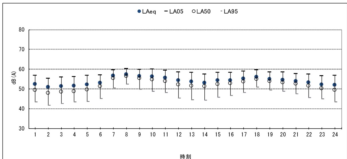
図Ⅱ-3.3 騒音レベル経時変化
