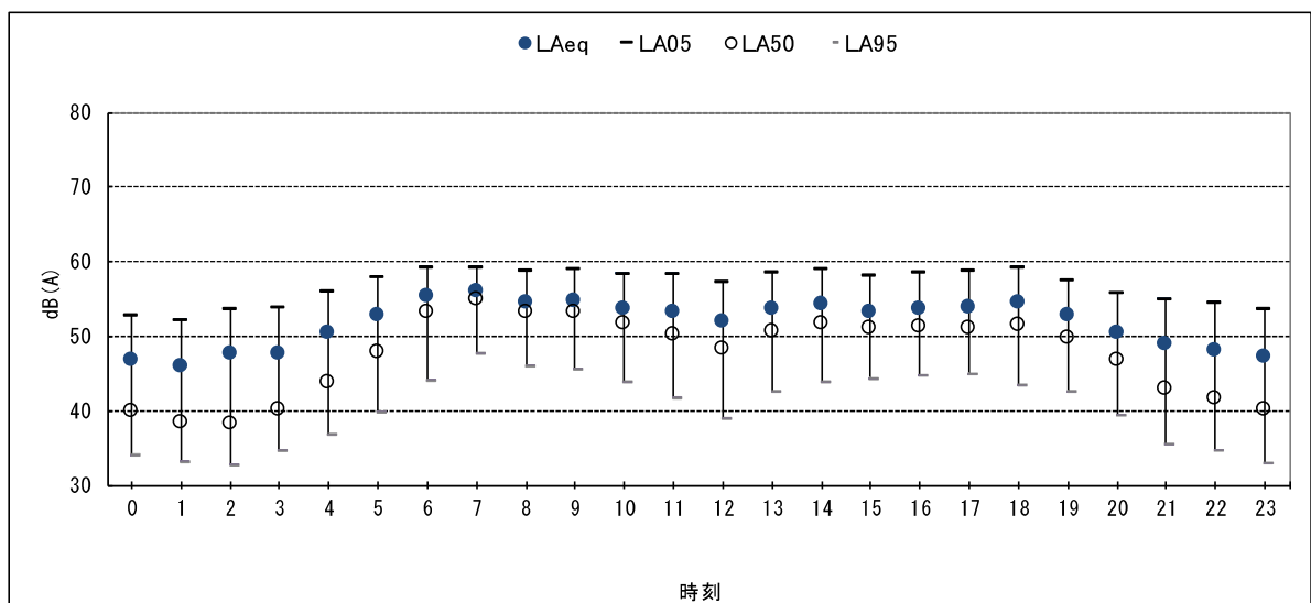
図Ⅱ-3.2 騒音レベル経時変化
