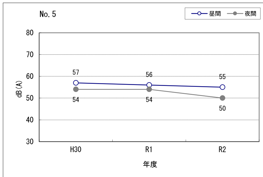
図Ⅱ-5.3 等価騒音レベルの経年変化（No. 5）
