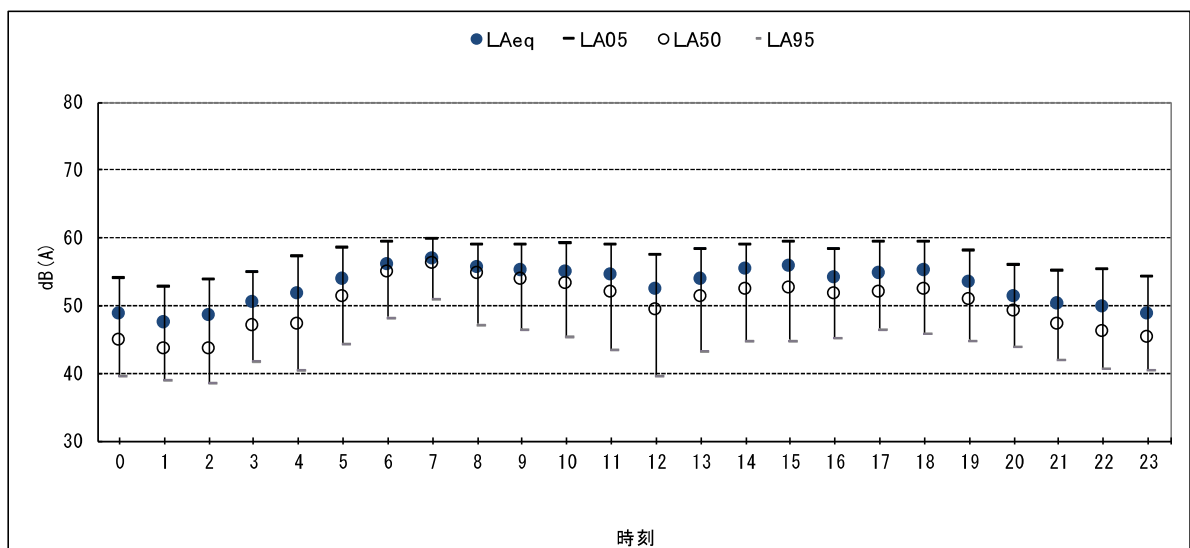
図Ⅱ-3.3 騒音レベル経時変化
