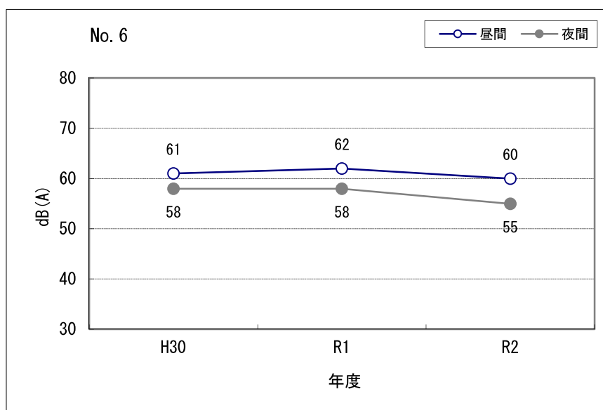
図Ⅱ-5.4 等価騒音レベルの経年変化（No. 6）
