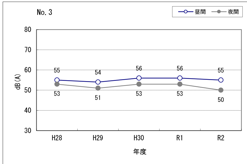
図Ⅱ-5.1 等価騒音レベルの経年変化（No. 3）
