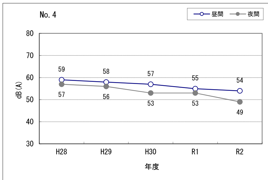
図Ⅱ-5.2 等価騒音レベルの経年変化（No. 4）
