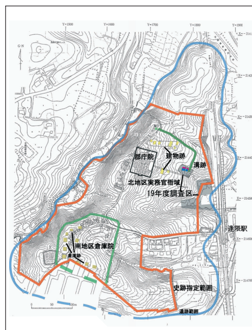
三十三間堂官衙遺跡全体図
