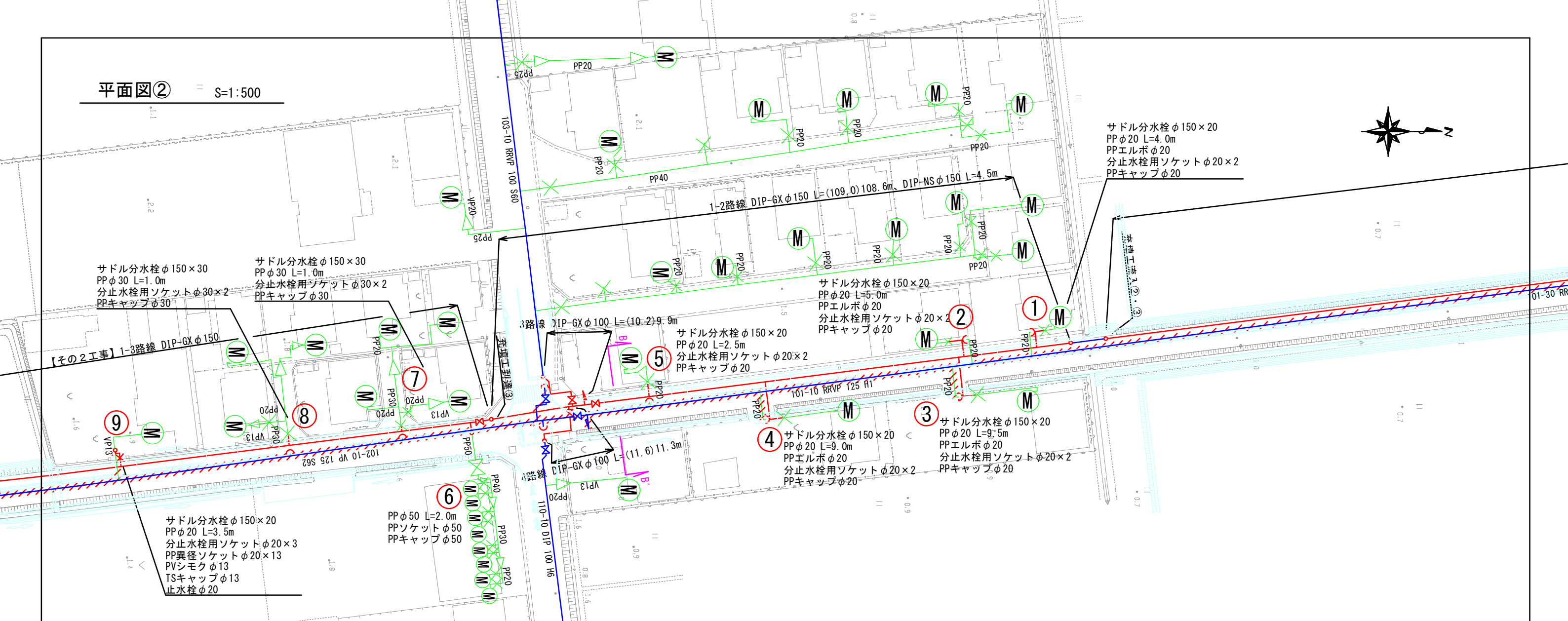
充填工詳細図 S=1:X RR-VPφ125 L=410.0m
