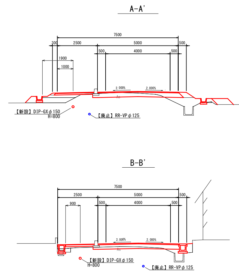
横断面 S=1:100
