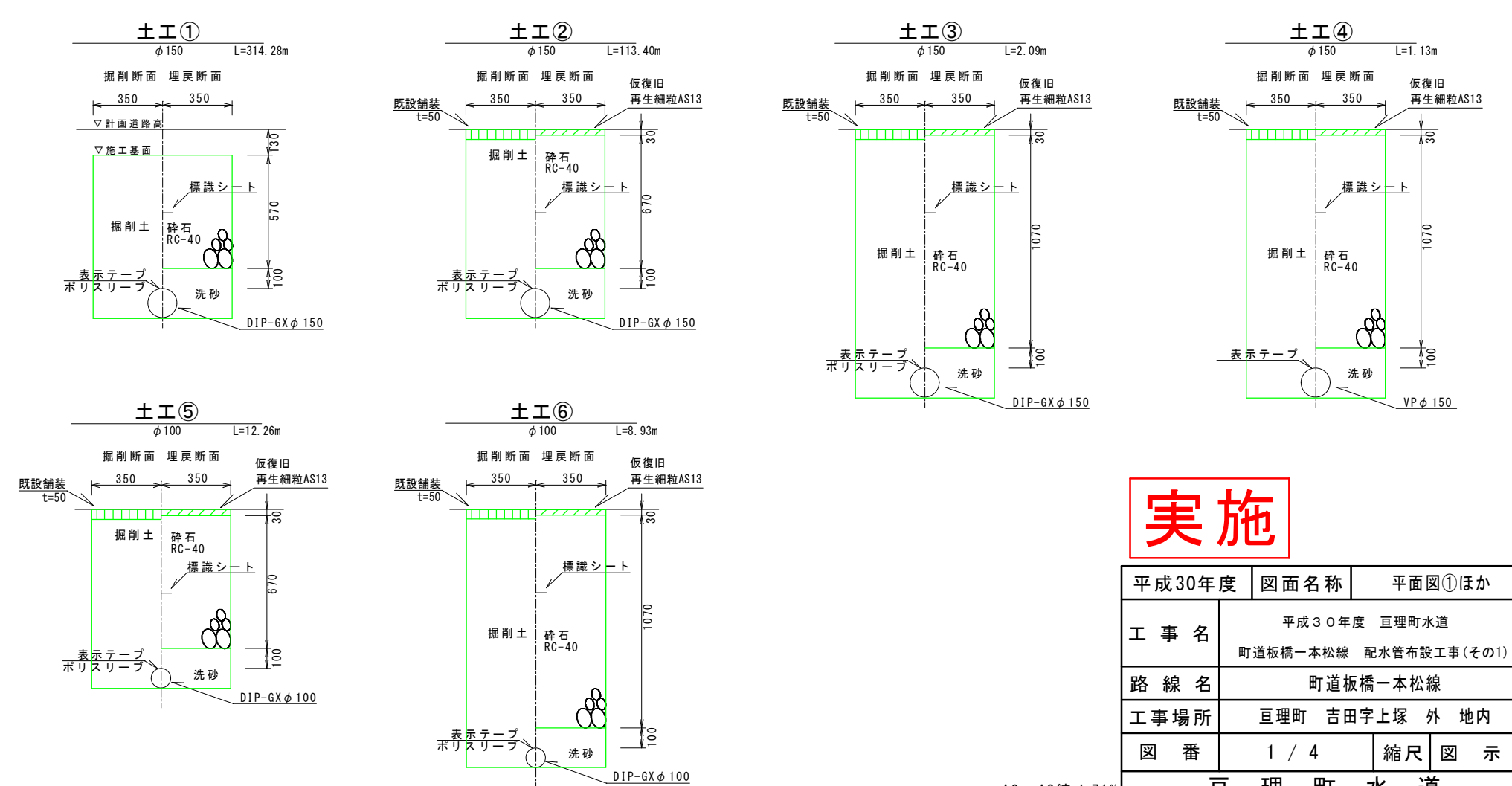
土工標準図 S=1:100
