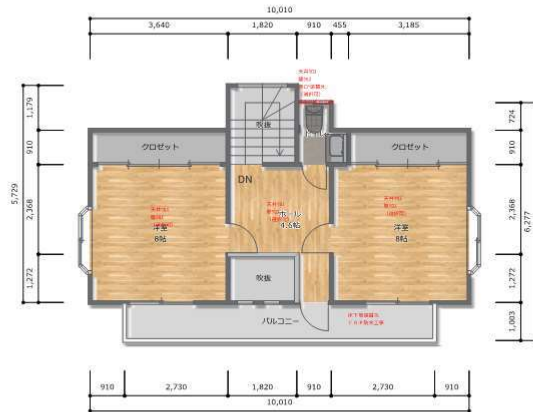
2階縮尺 1/100
