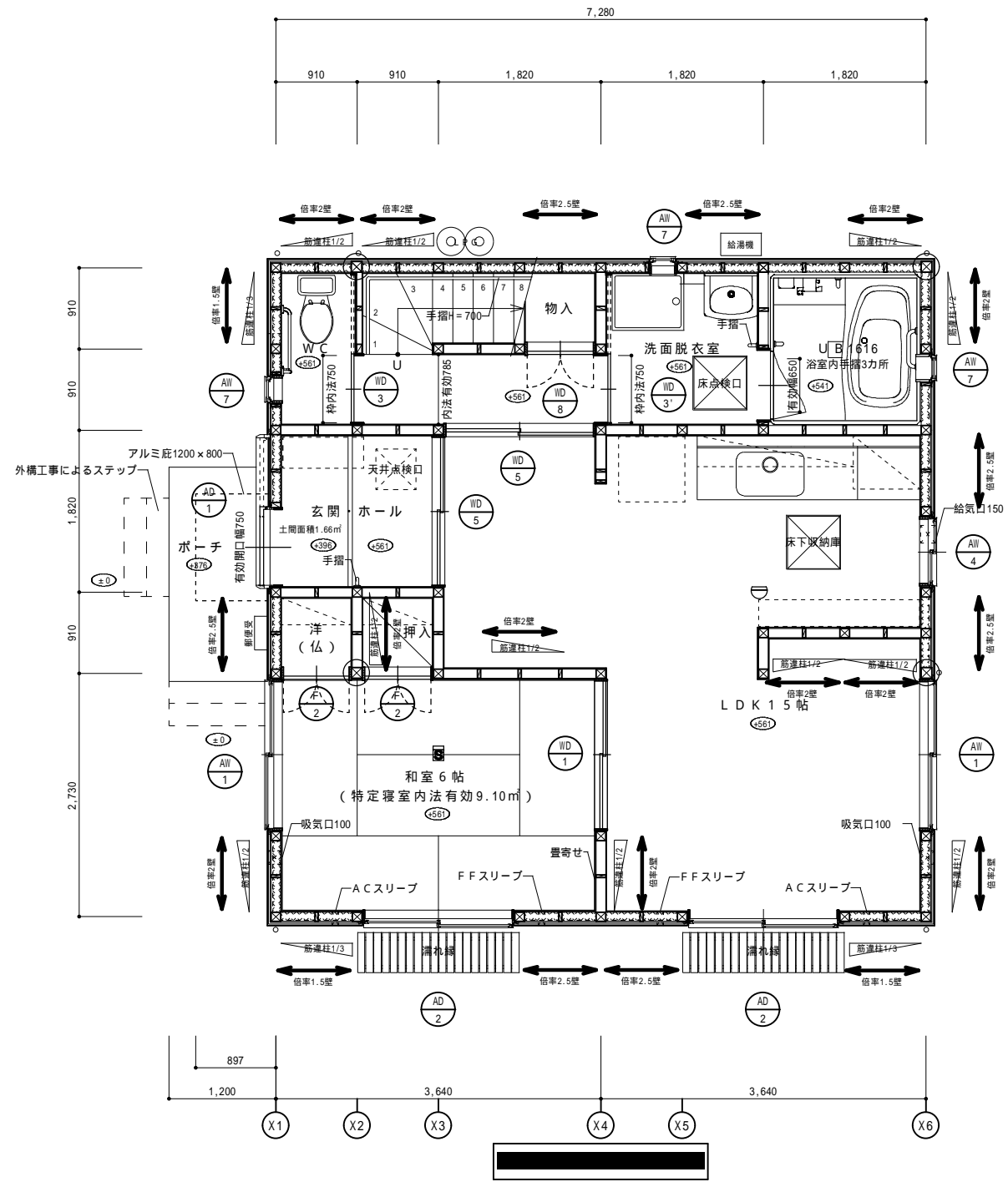
1階平面図
