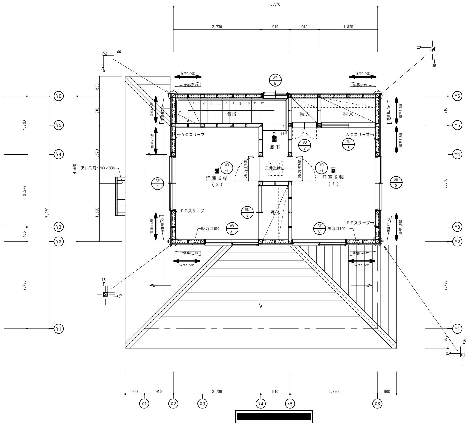
2階平面図
